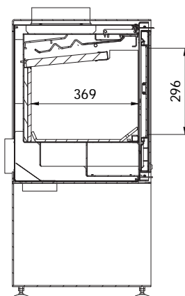
C-C ( 1 : 10 )
