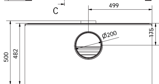
D-D ( 1 : 10 )
