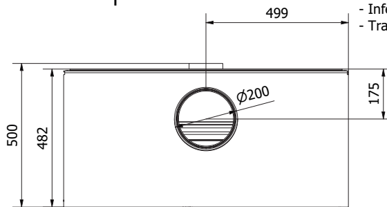
G-G ( 1 : 10 )
