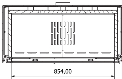
G-G ( 1 : 10 )
