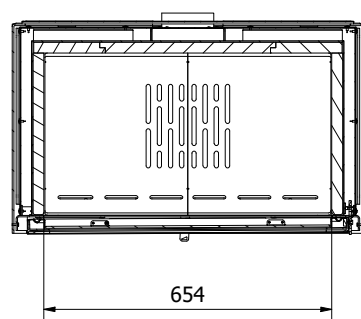
D-D ( 1 : 10 )
