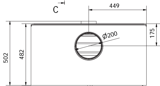
D-D (1 : 10)
