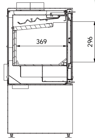
C-C (1 : 10)
